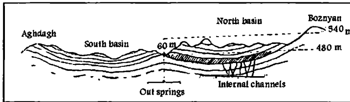
شپوهی ٤٦- نیوه پرو (پرو فیل) ی پیکهانه بهردیه کانی نزیک سهرچاوه نهوتیه کان.
