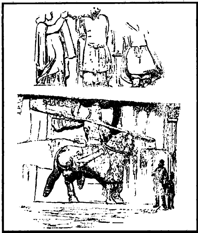
شێوه‌ی 04- هه‌لکه‌ندراوه‌کانی تاق و هسان
